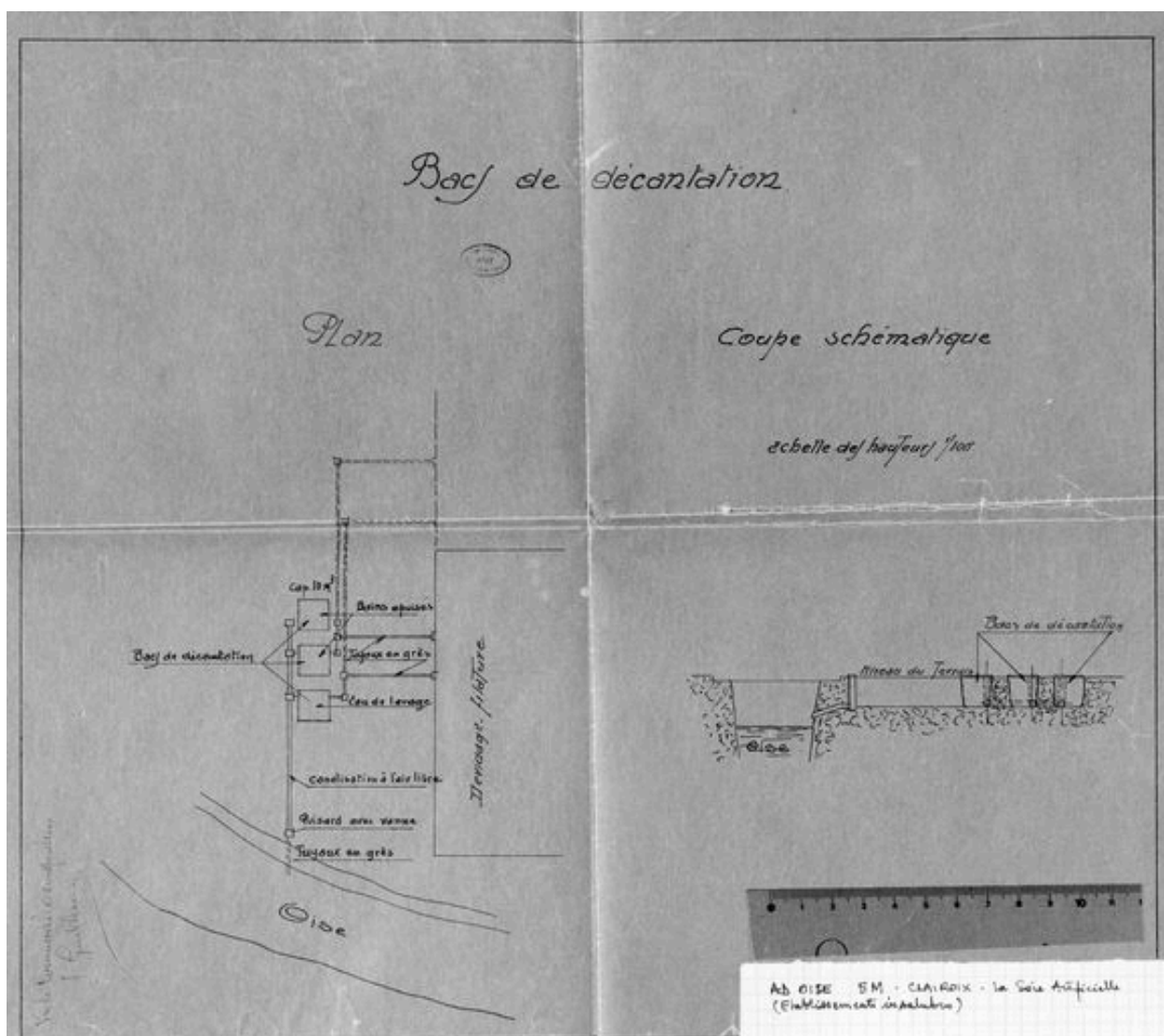
Coupe et plan des bacs de décantation (AD Oise ; Mp 2444).
