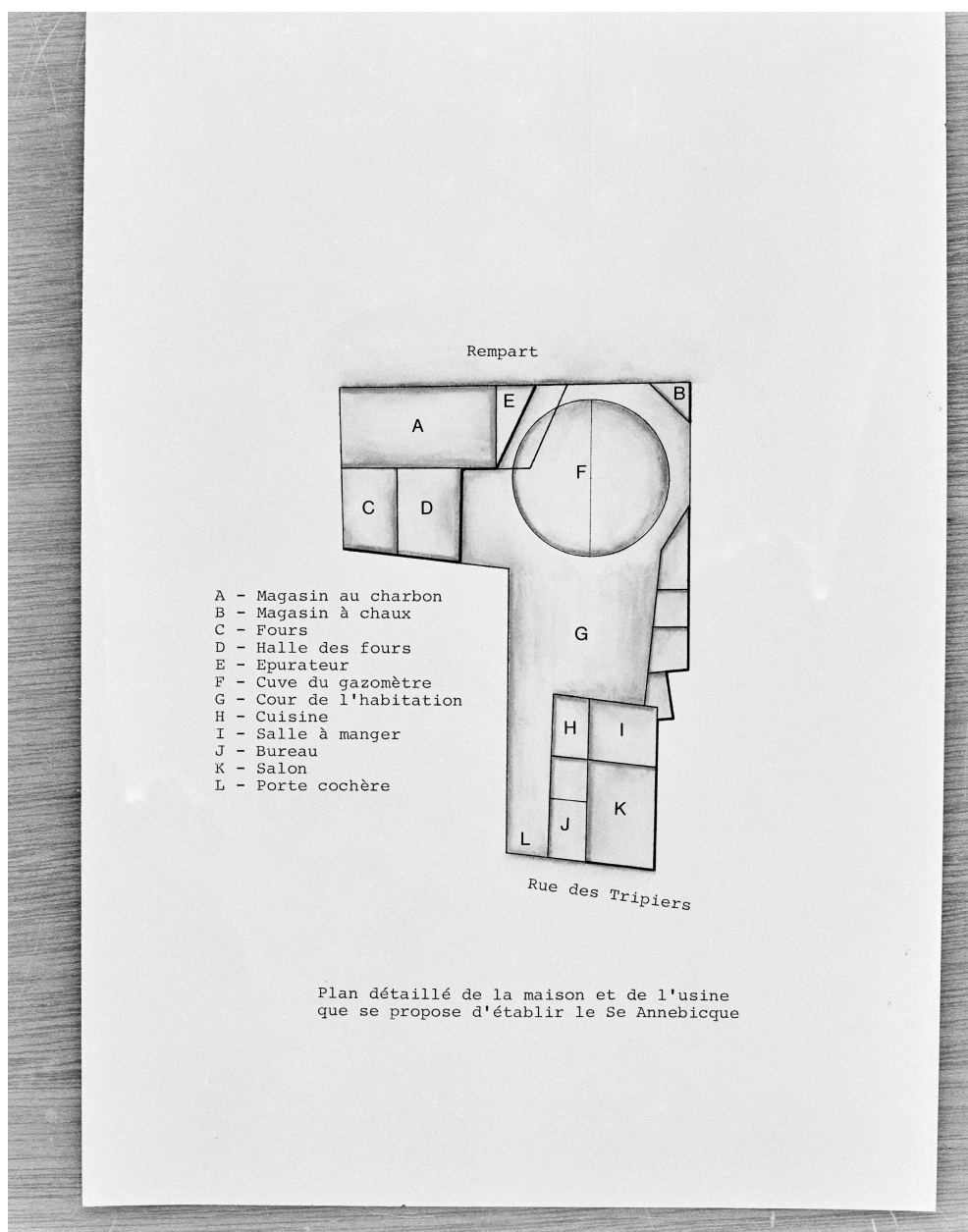
Plan détaillé de la maison et de l'usine que se propose d'établir le sieur Annebicque en 1845-1846 (AD Pas-de-Calais, M 3113).
