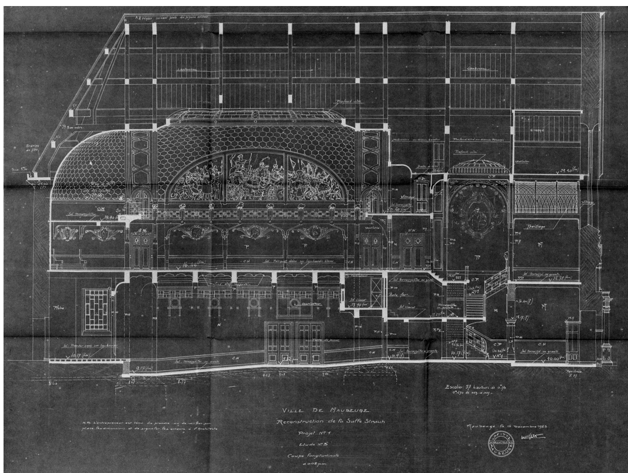
Projet n° 1 de reconstruction de la salle Sthrau, coupe longitudinale (avec décor). Plan n° A 786, Maubeuge, 16 décembre 1923, par Jean et Henri Lafitte (ingénieurs-architectes) (?) (AD Nord O396/682).
