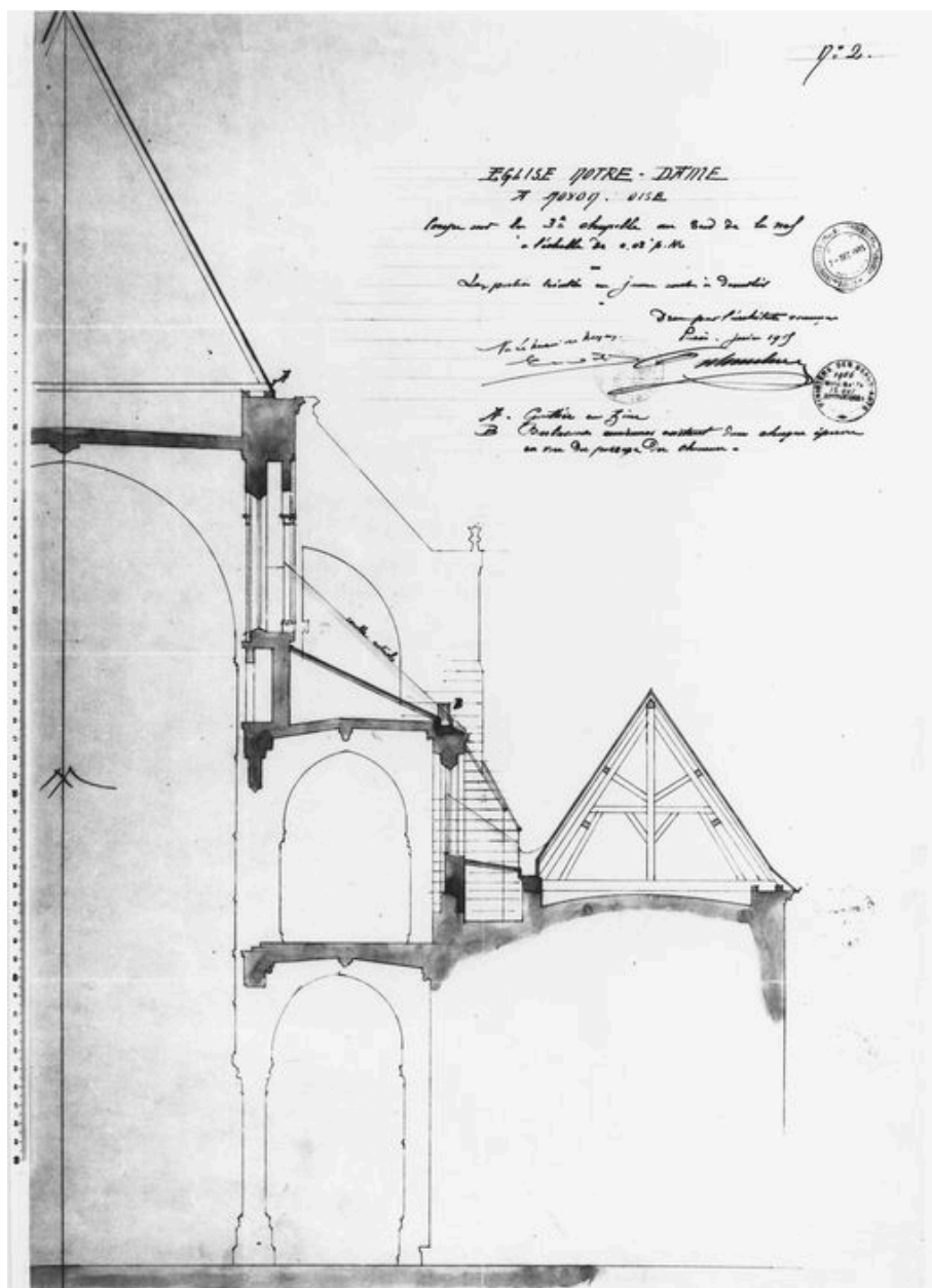
3e chapelle sud de la nef. Coupe par Selmersheim, 1905.
