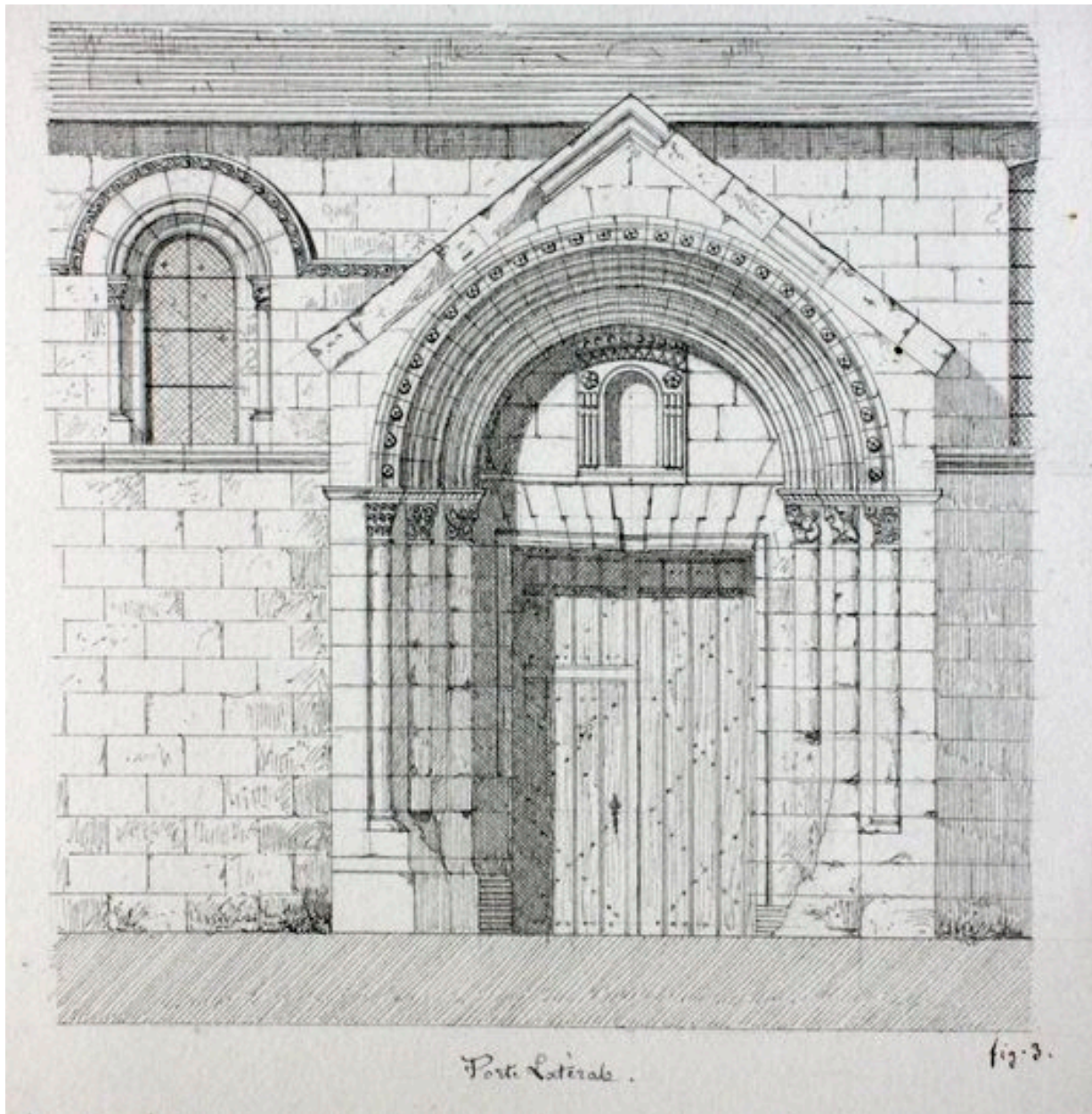
Portail latéral sud par Hyacinthe Dusevel, 1842 (AMH, Médiathèque de l'Architecture du Patrimoine. Berteaucourt-lès-Dames ; 80/81).
