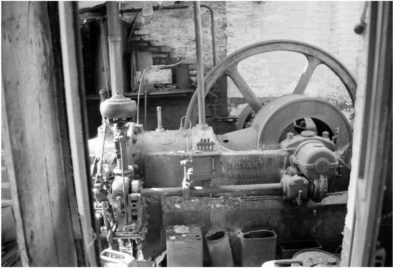
Moteur à pistons à combustion (machine à pression d'huile) : vue de profil.
