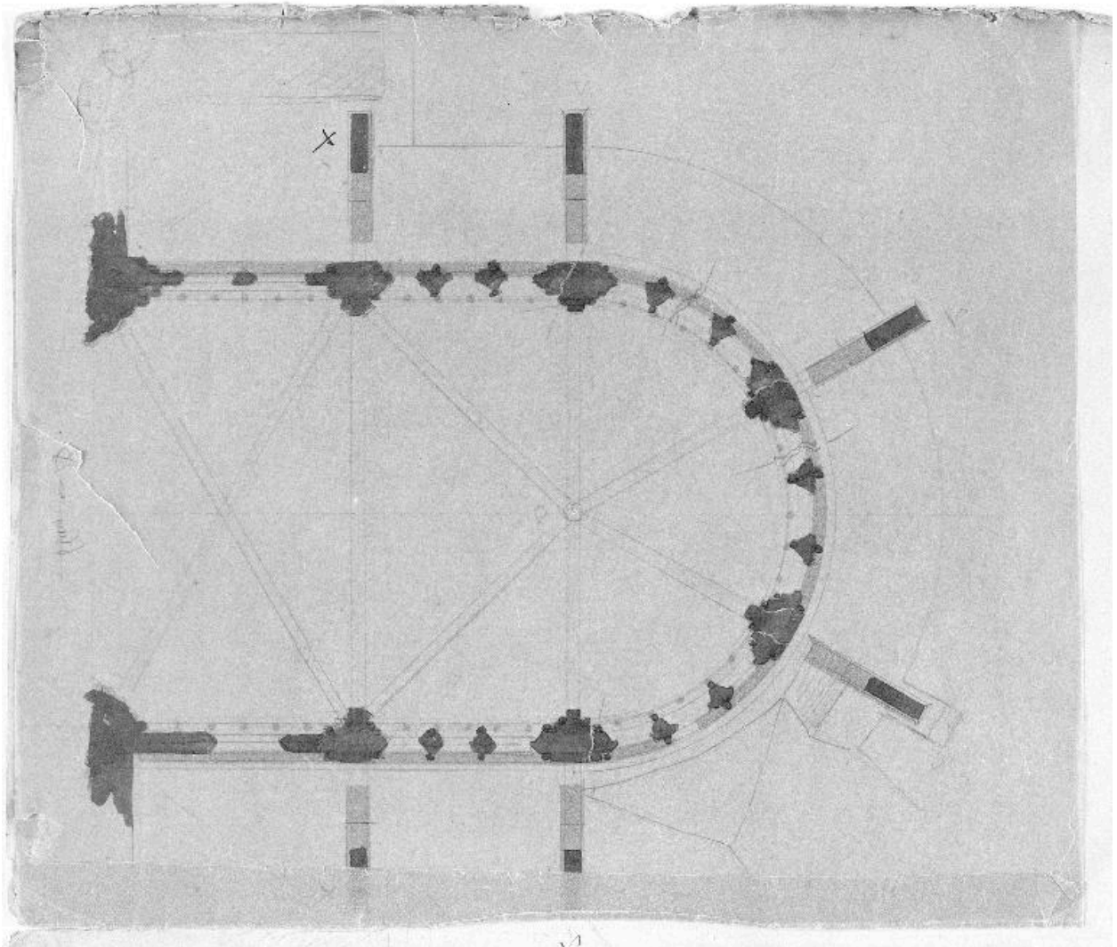
Plan du quatrième niveau du bras sud du transept, dessiné vers 1875 par un architecte diocésain dans le cadre de sa restauration (AN F 19 7888).
