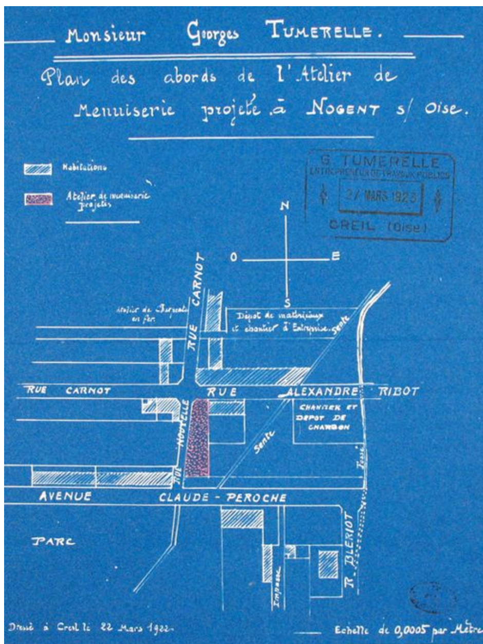
Plan des abords de la menuiserie Tumerelle, 1922 (AD Oise ; 5Mp2519).
