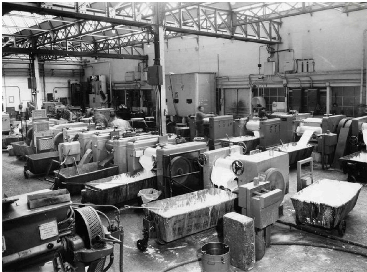
Broyeuses trois cylindres, vers 1950 (archives d'entreprise).
