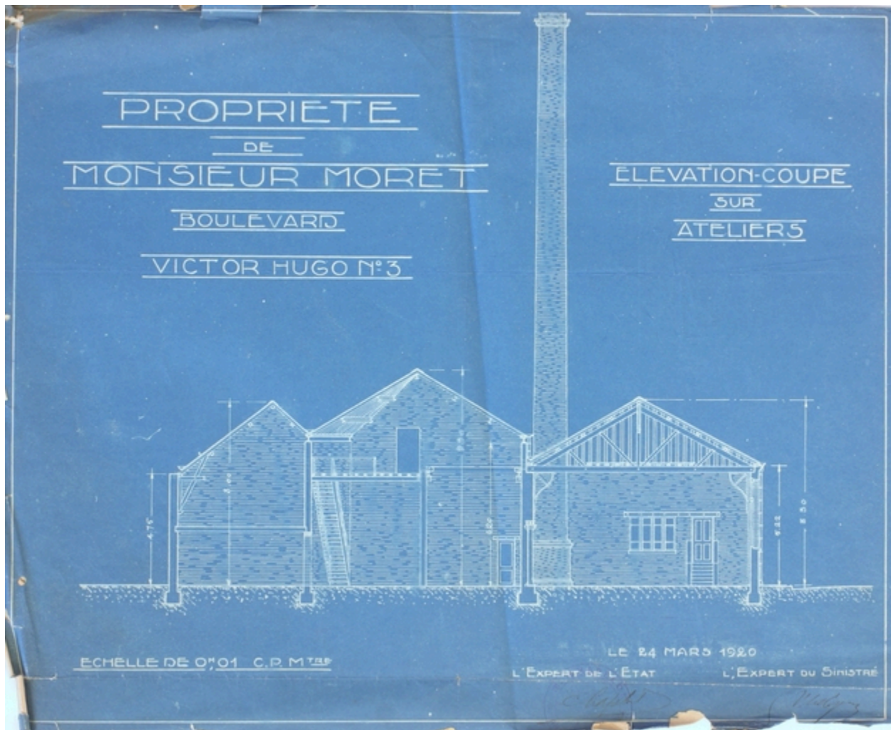
Elévation et coupe des ateliers, avant 1914, par Malgras-Delmas (AD Aisne).
