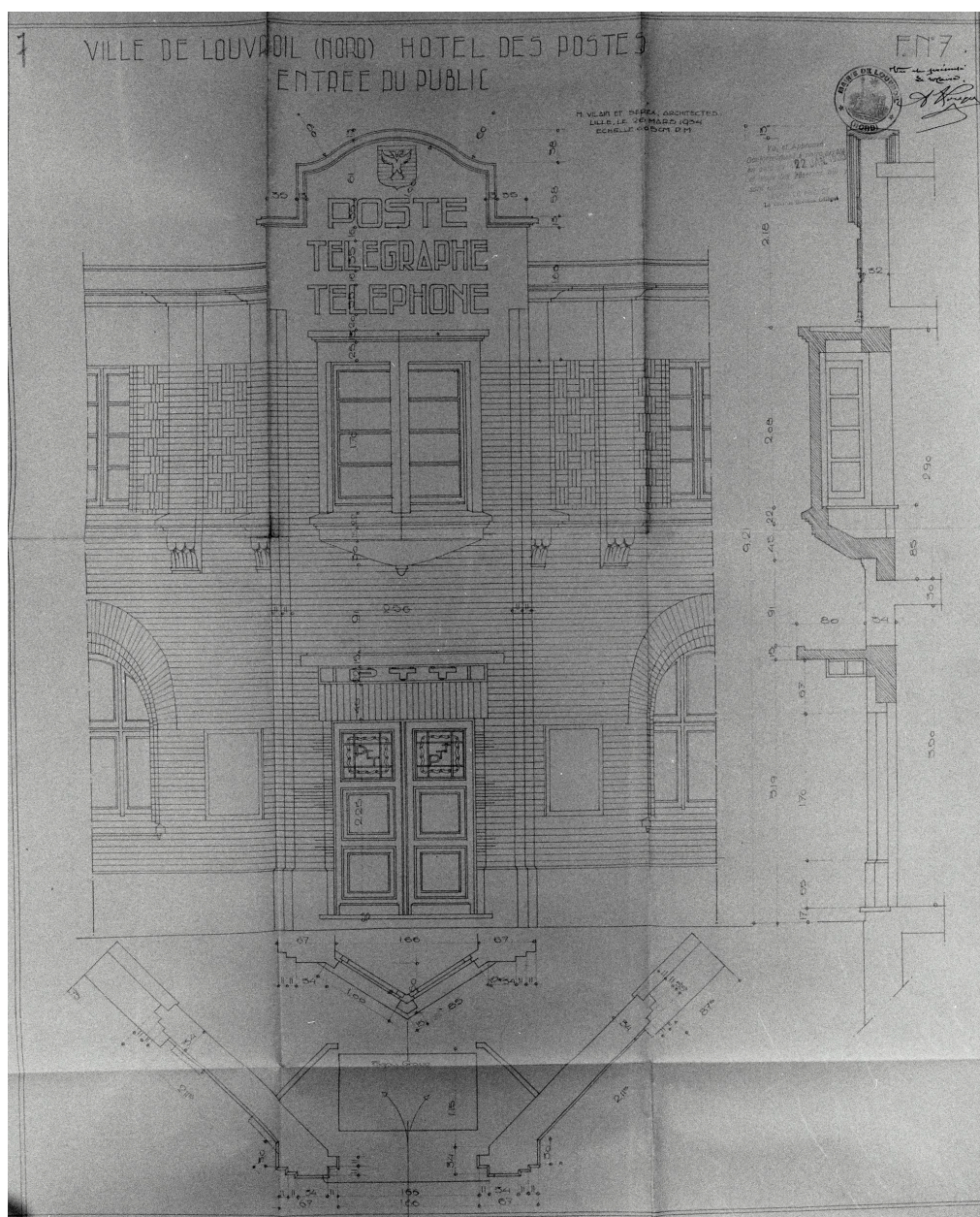
Élévation antérieure de l'entrée principale par Vilain (architecte) et Serex (architecte), 1934 (AD Nord ; O371/157).
