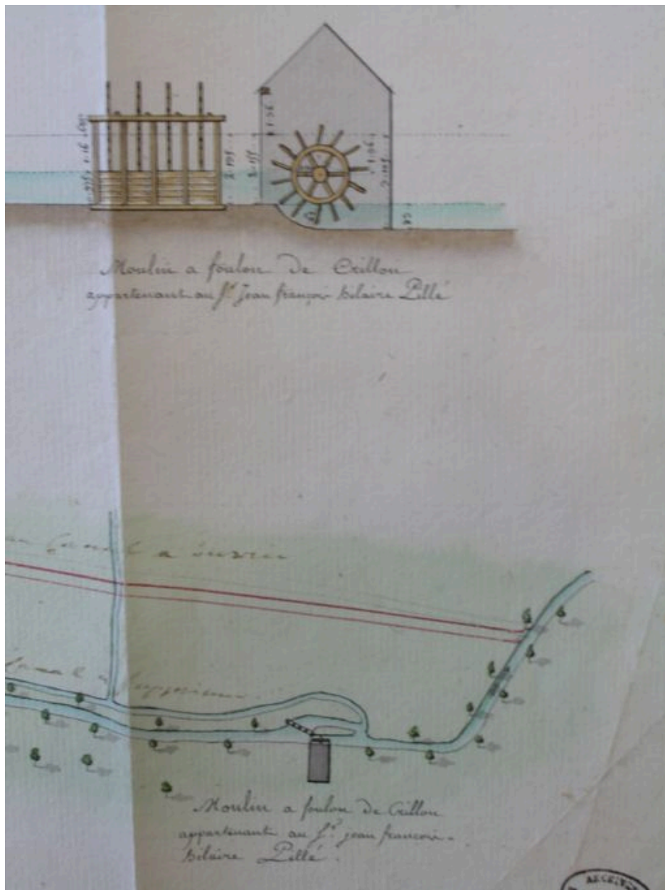
Plan et profil du moulin à foulon de Crillon, extrait du plan de la rivière du Thérain entre les moulins à foulon Pillet de Martincourt et celui de Crillon, 15 juin 1809.
