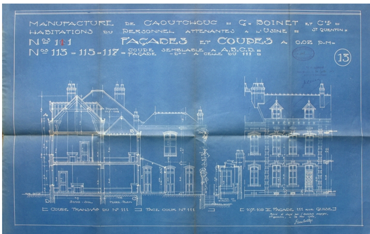
Coupe et façade antérieure d'un logement rue de Guise, par Le Bot, 1920 (AC Saint-Quentin).
