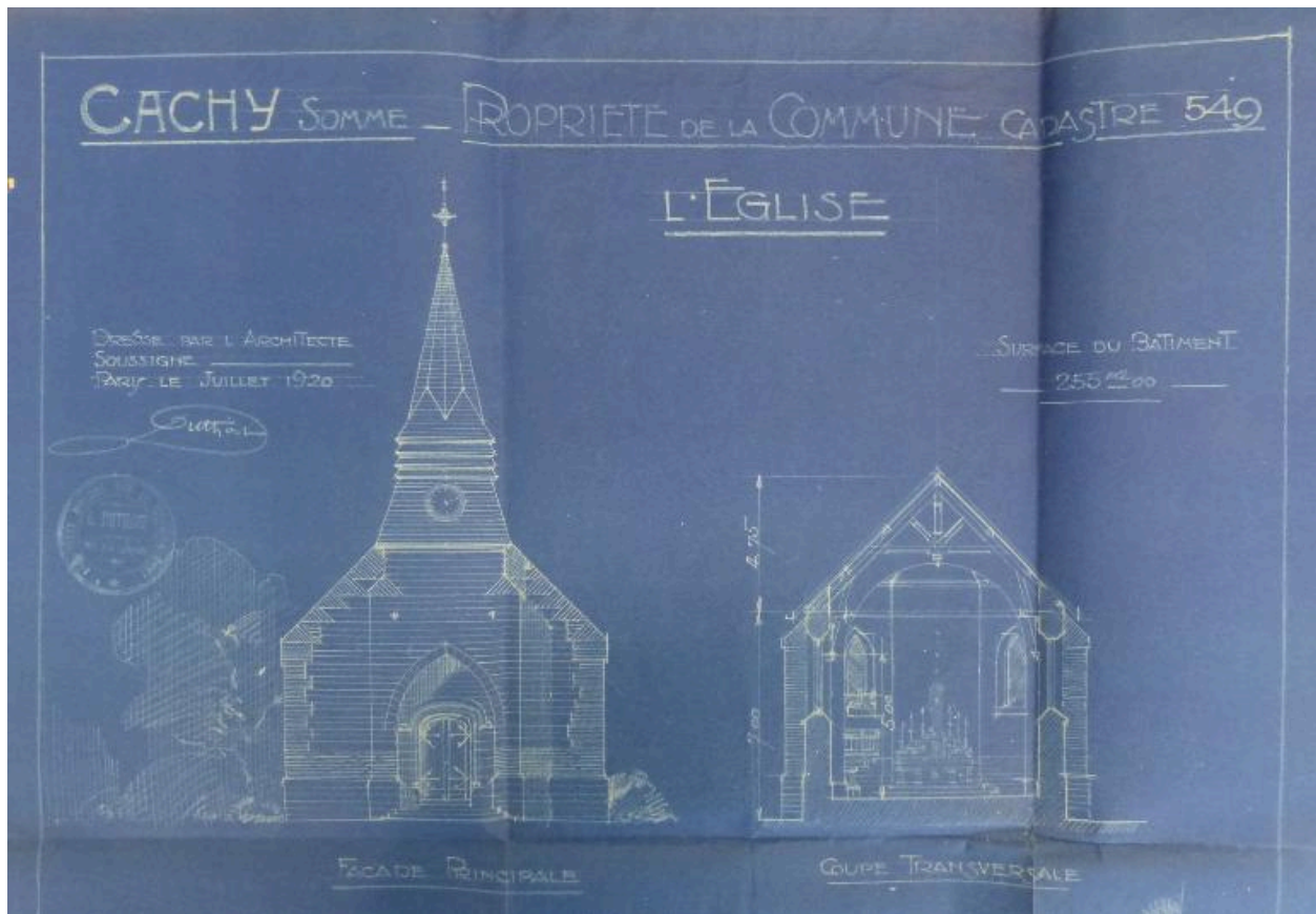
Cachy - Somme. [Ancienne] église, élévation et coupe, Louis Duthoit, 1920 (AD Somme ; 10 R 263).
