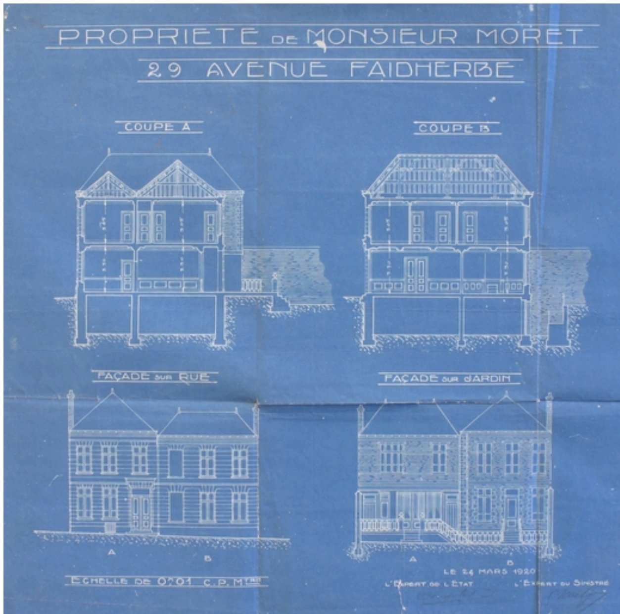
Coupes et élévations du logement patronal avant 1914, par Malgras-Delmas (AD Aisne).
