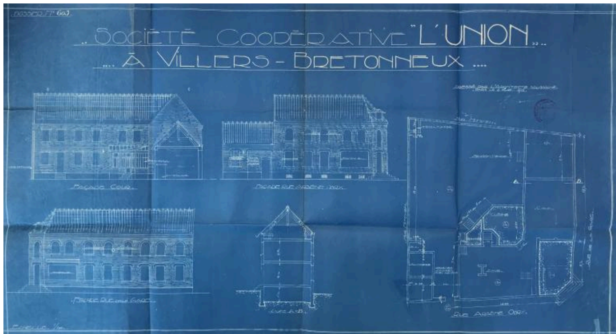
Société coopérative de l'Union à Villers-Bretonneux. Plans, élévations et coupe, 1922 (AD Somme ; 10R 1250).
