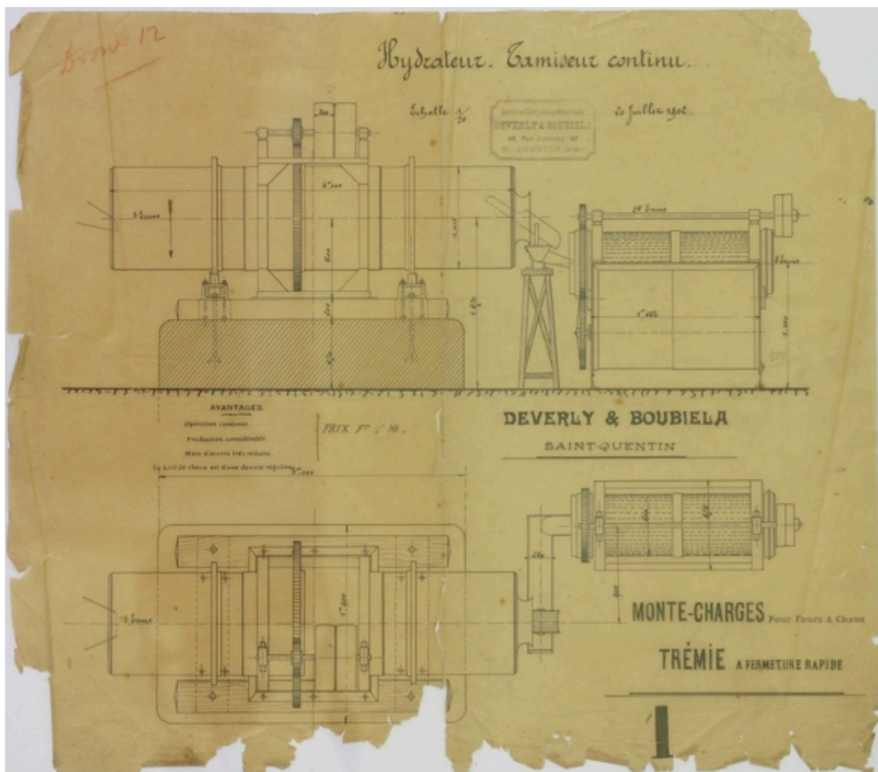
Plan d'un hydrateur-tamiseur continu construit par les ateliers Boubiéla et Deverly en 1902 (AP).
