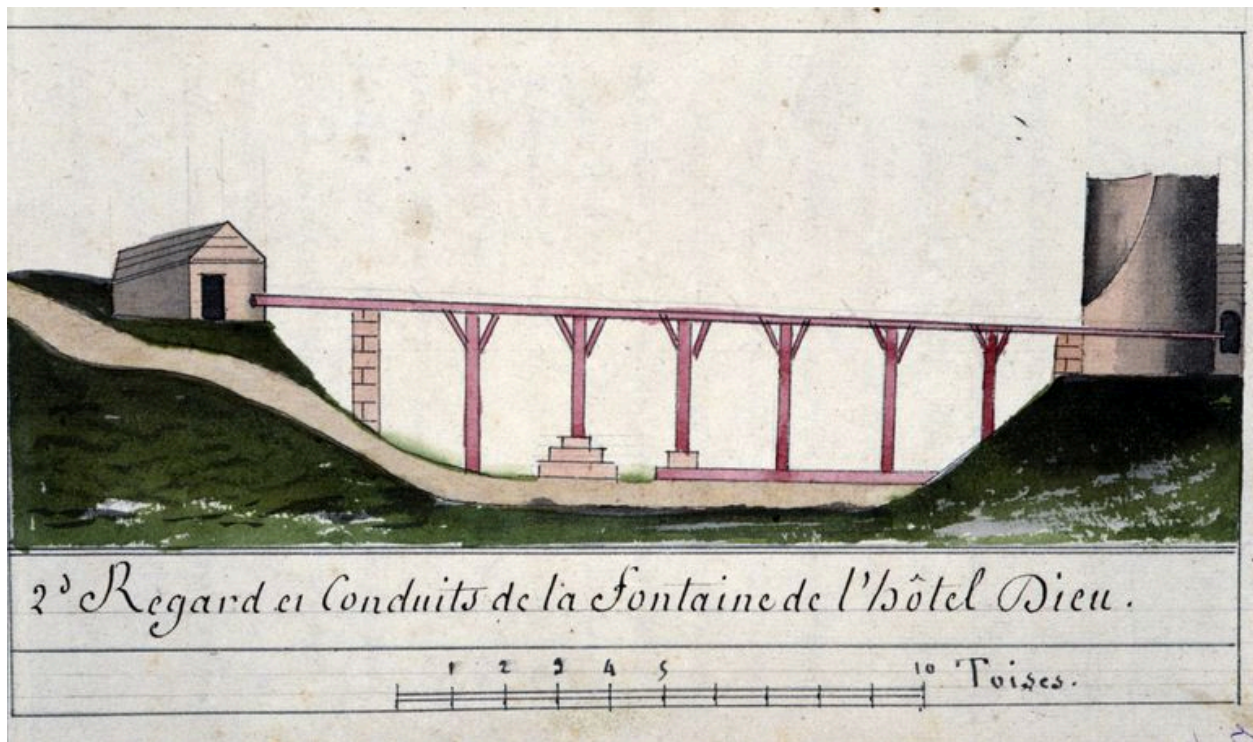
Regard et conduits de la fontaine de l'hôtel Dieu, vers 1816 (BM Compiègne ; fonds Léré, V. de C. n 58 f 289).
