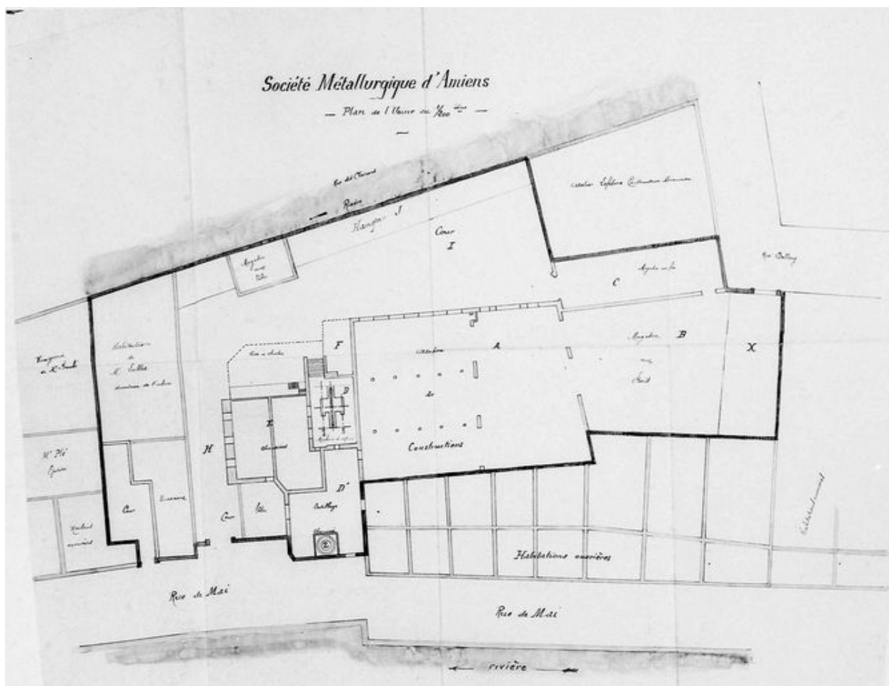
Plan de l'usine de la société métallurgique d'Amiens, dessin vers 1901 (AD Somme ; M 81740).
