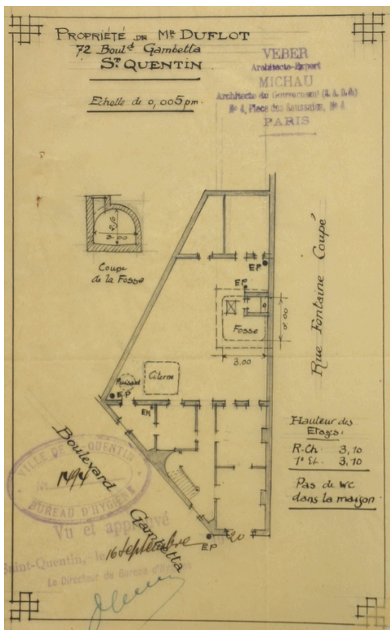
Plan du rez-de-chaussée du magasin implanté à l'angle de la rue Fontaine-Coupé et du boulevard Gambetta, par Veber et Michau, 1920 (AC Saint-Quentin).
