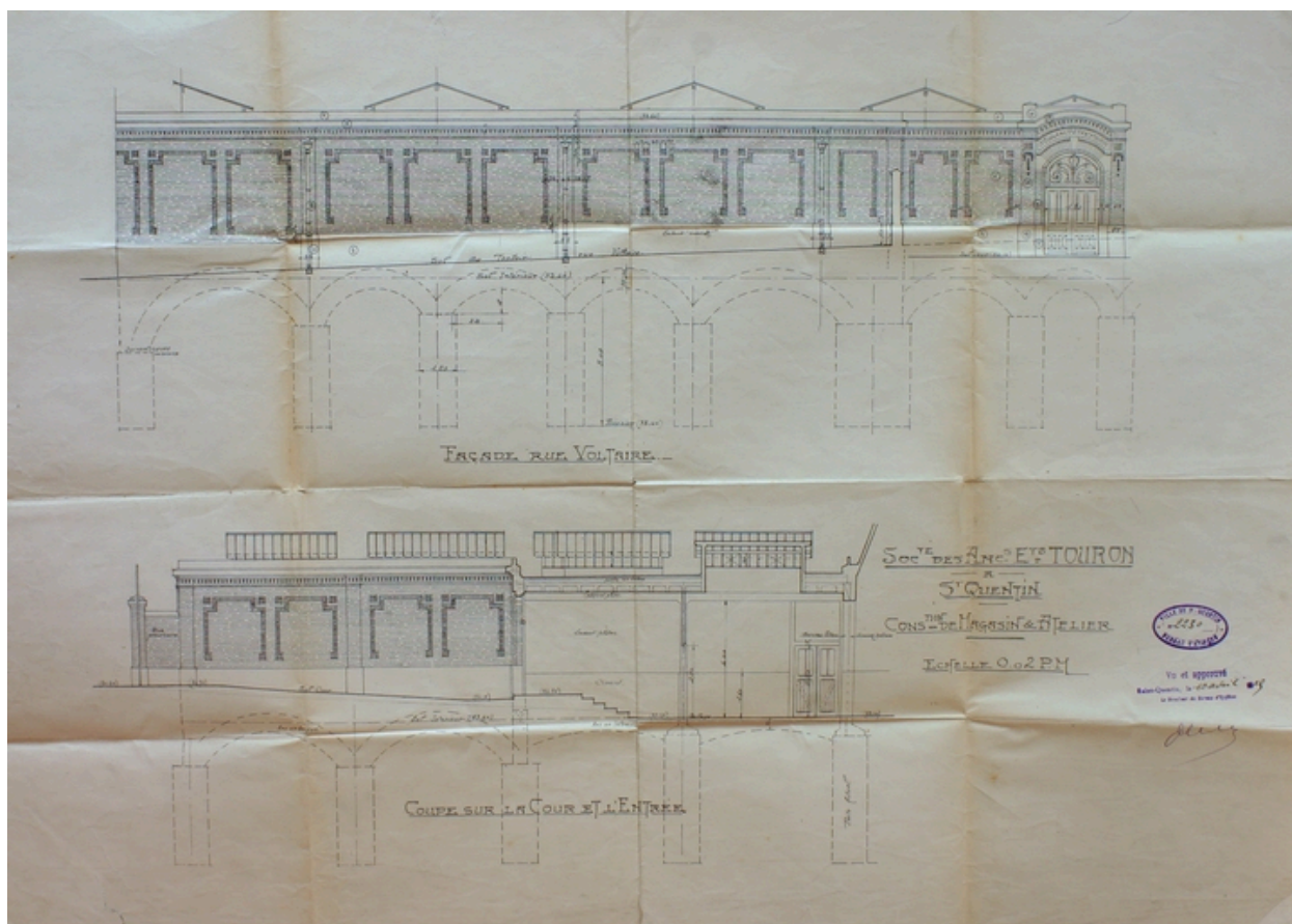
Plans d'agrandissement de la filature, par Nalet (arch.), 1925 (AC Saint-Quentin).
