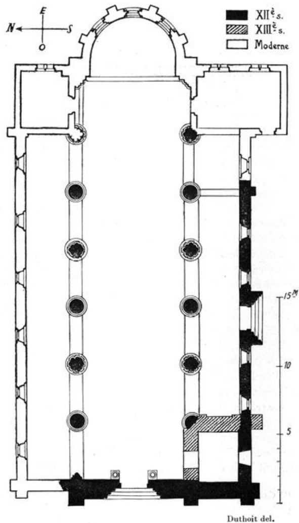
PLAN DE L'ÉGLISE DE BERTEAUCOURT-LES-DAMES
