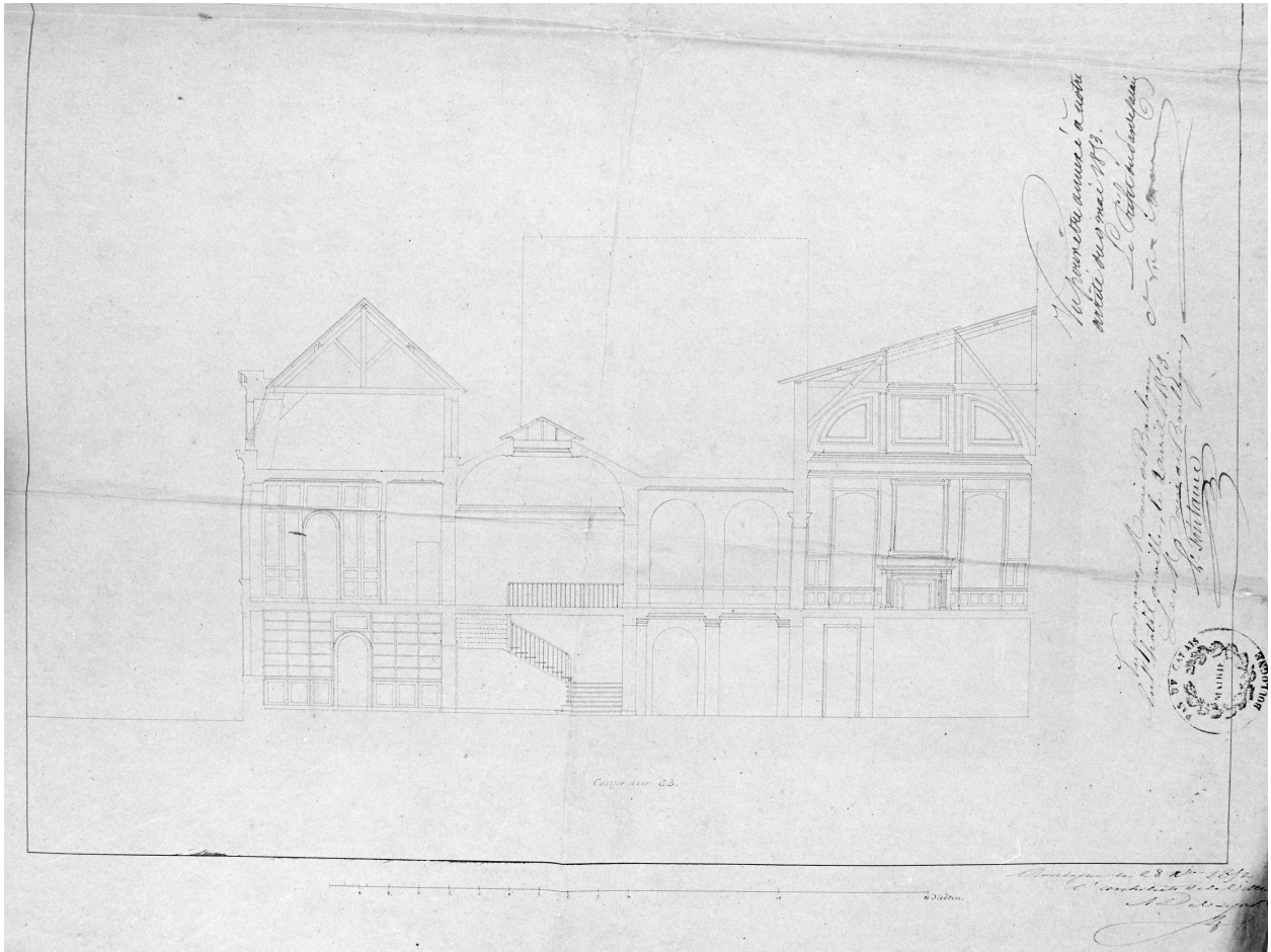
Projet de 1852, signé Debayser ; coupe. A.D. Pas-de-Calais, 2 0 - 1121.
