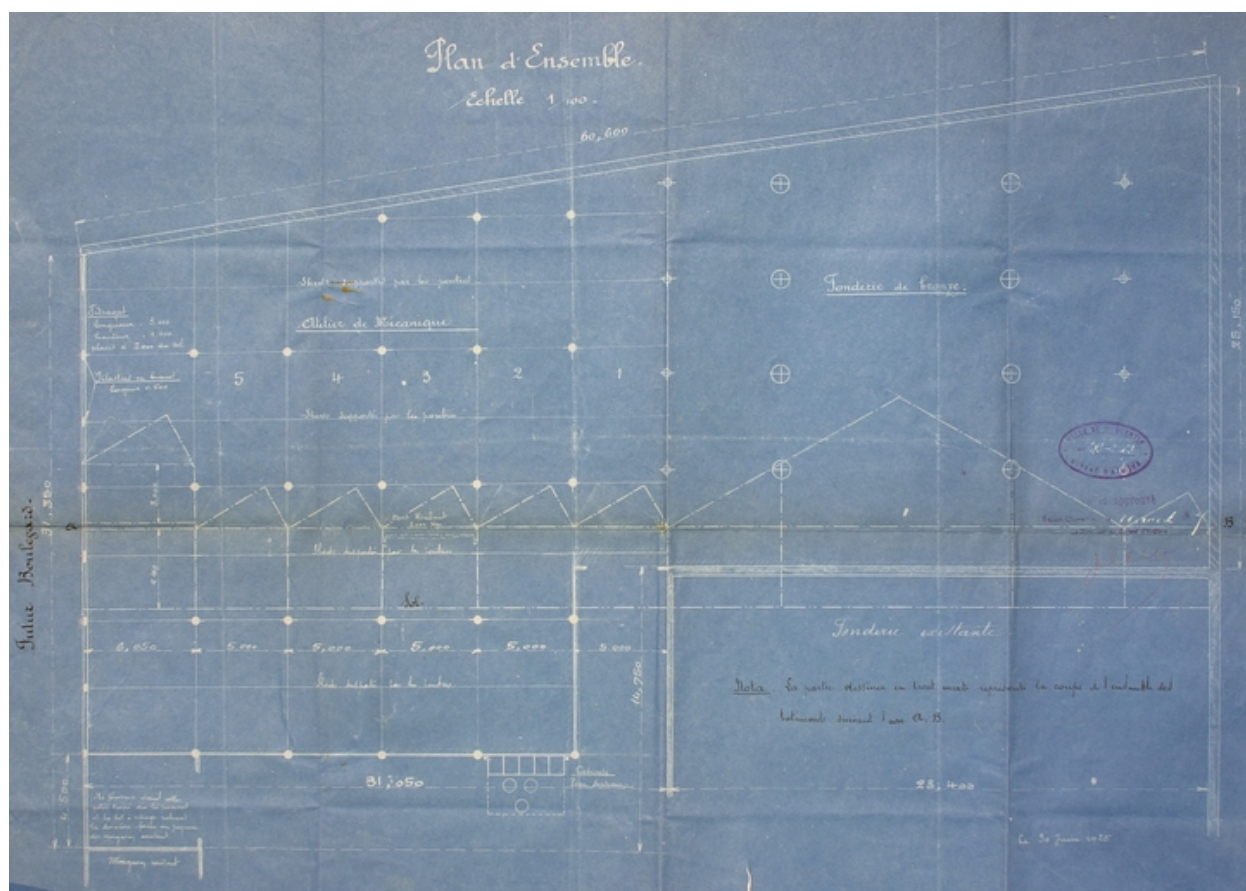
Plan d'un nouvel atelier, 1925 (AC Saint-Quentin).
