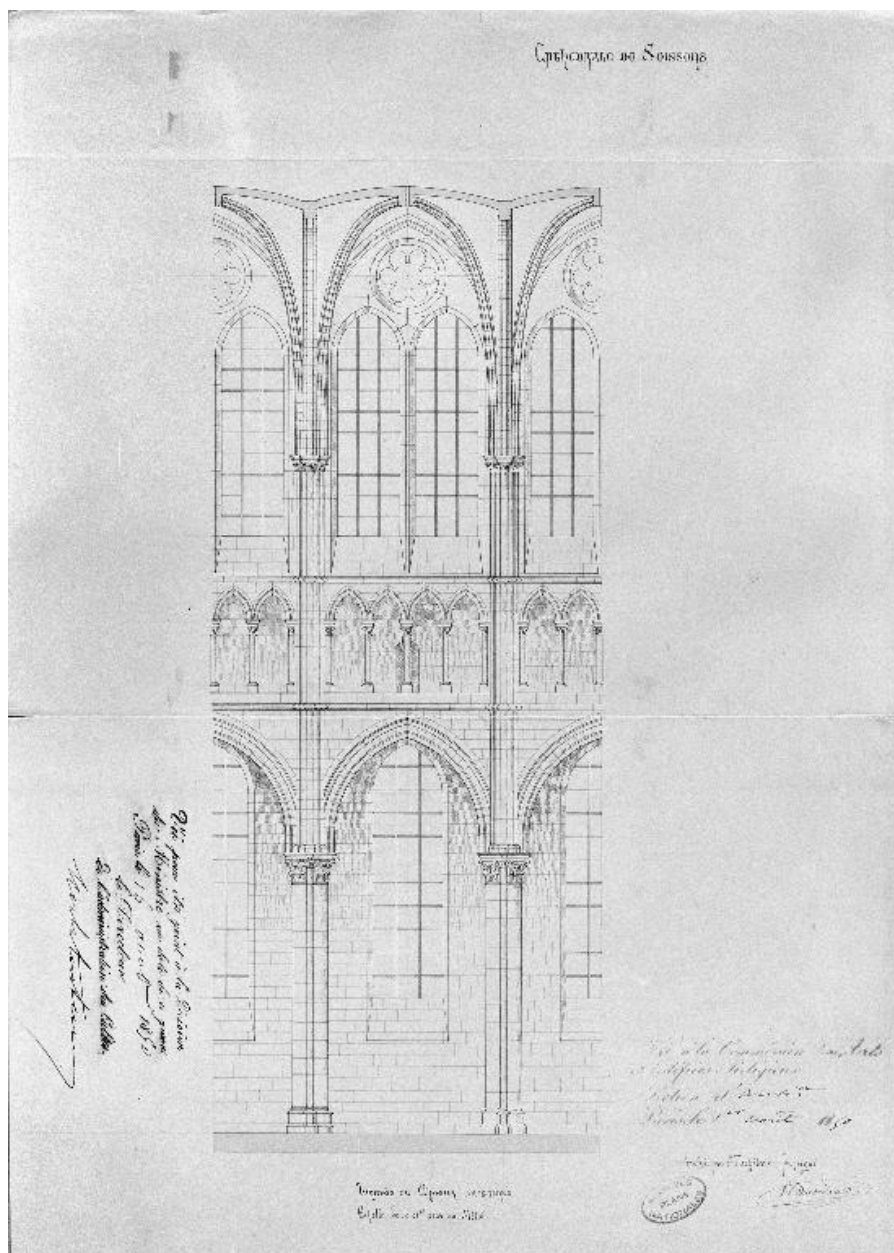
Élévation intérieure d'une travée du chœur restaurée, dessinée par l'architecte Émile Boeswillwald en 1850 (AN : F 19 7887).
