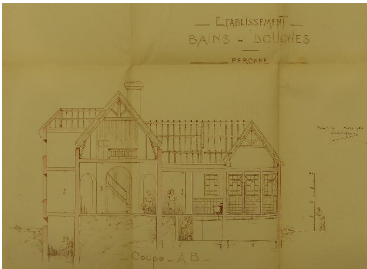
Caisse d'Epargne de Péronne. Etablissement de bains douches. Coupe, Marcel Debefaudé entrepreneur, 1924 (AD Somme ; 10R 1018).
