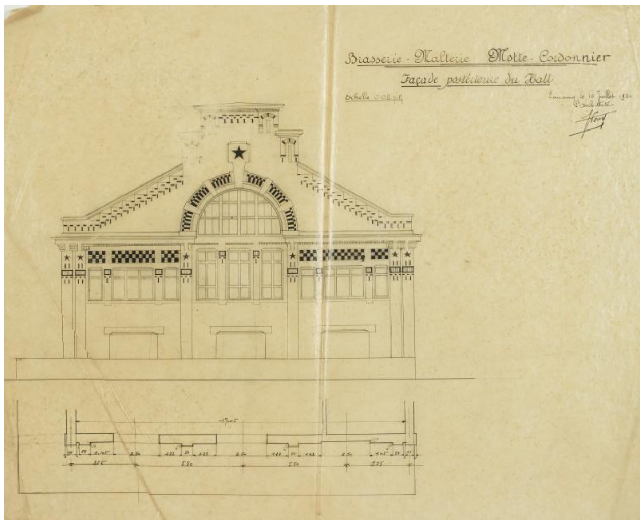
Brasserie-Malterie Motte-Cordonnier. Façade postérieure du hall. Coupe élévation par l'architecte Georges Forest, 16 juillet 1920 (coll. part. Motte).
