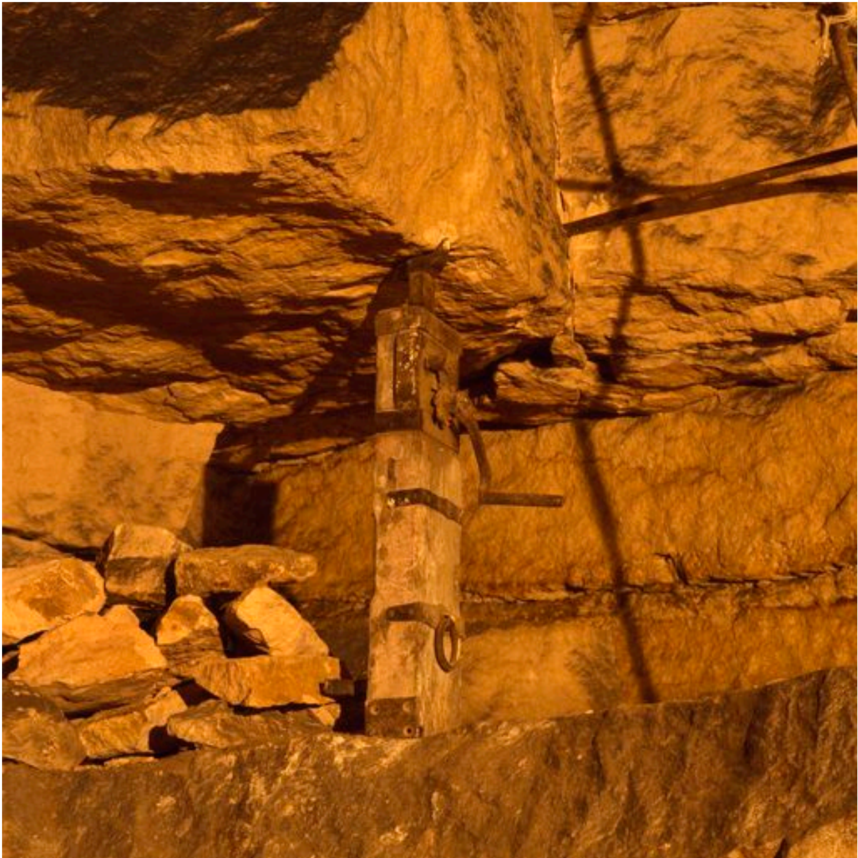
Soutènement d'une partie d'un bloc de pierre.
