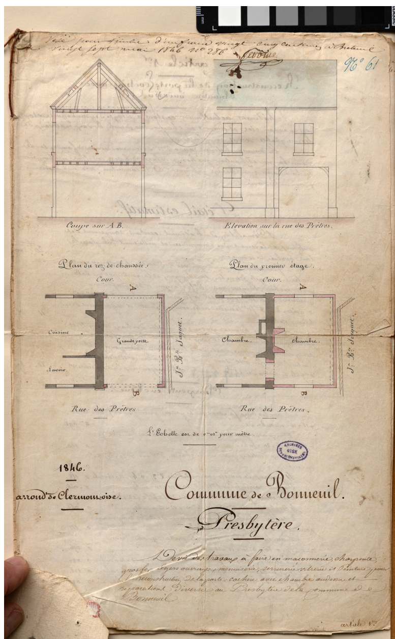
Plan du presbytère, 1846 (AD Oise).
