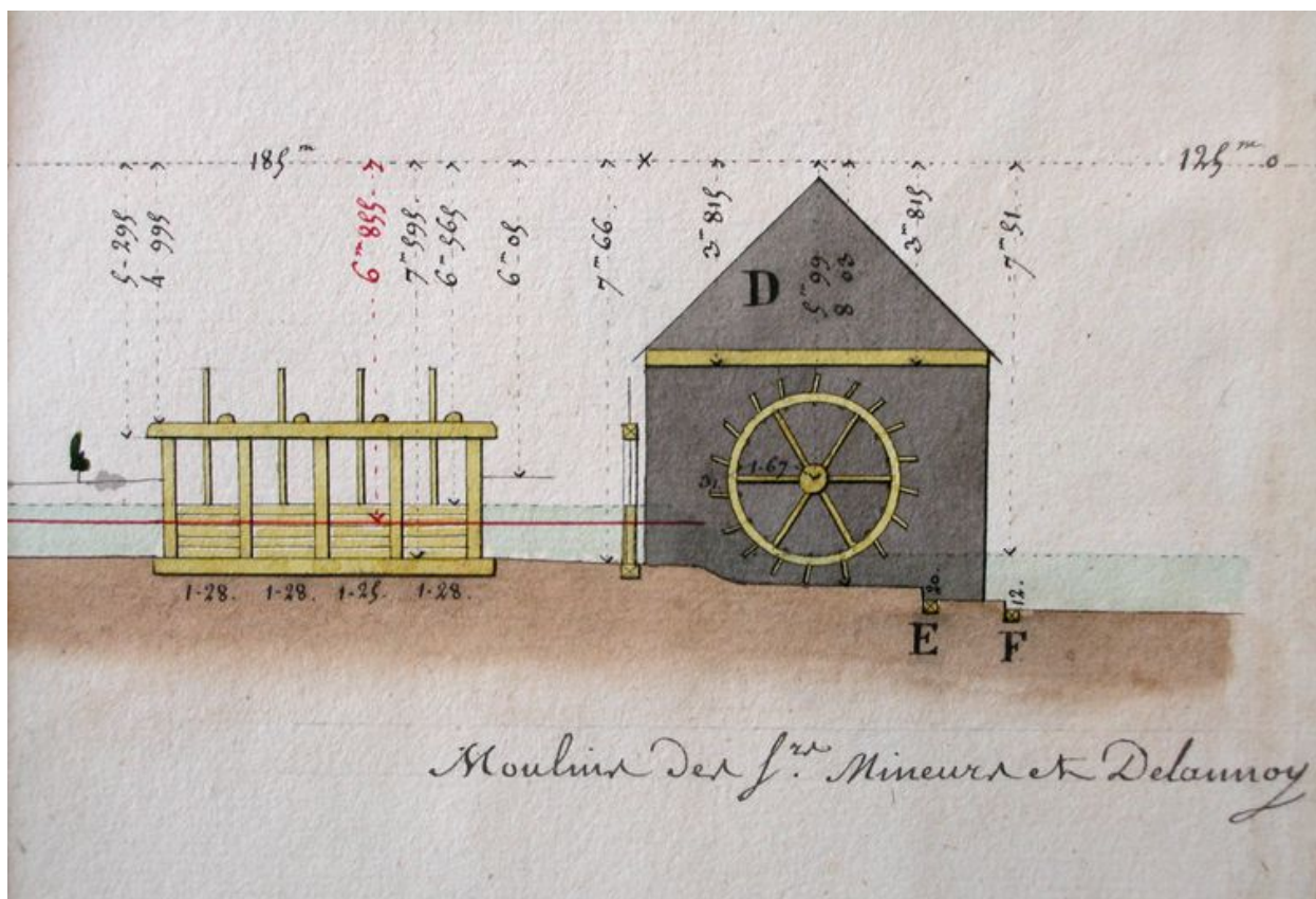
Profil du moulin à draps et à blé appartenant à Mineur et Delannoy, 1812.
