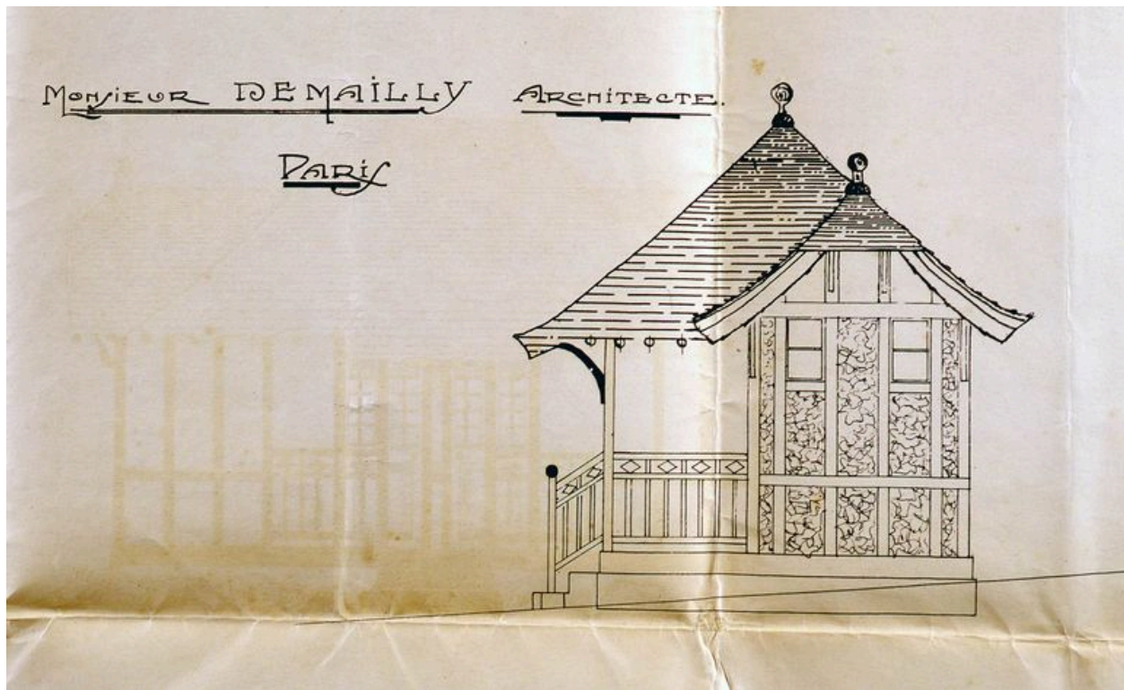
Élévation latérale, par Demailly architecte, 2e quart 20e siècle (AC Cayeux-sur-Mer).
