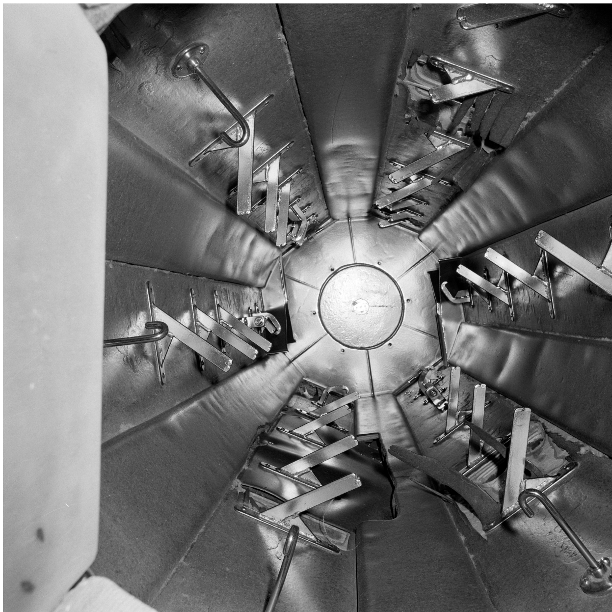
Tonneau de nettoyage des canettes. Vue intérieure.
