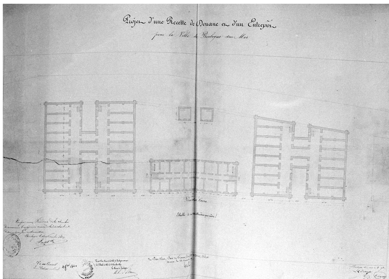
Douane, entrepôt public, plan du sous-sol, éch. 0,01 p.m. B.M. Boulogne-sur-Mer, ms 535 P. pl. 5.
