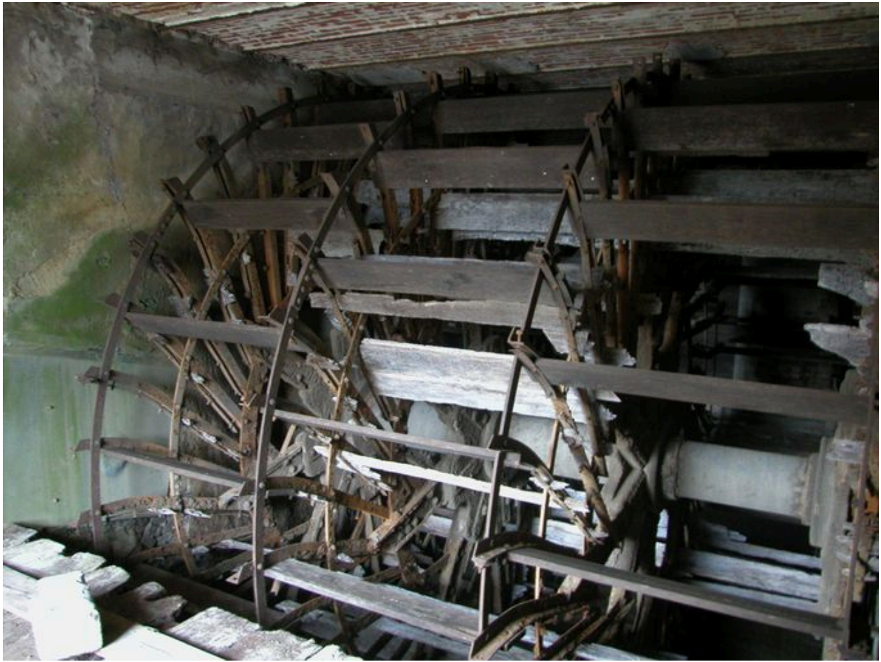
La roue hydraulique, vue de trois-quarts.
