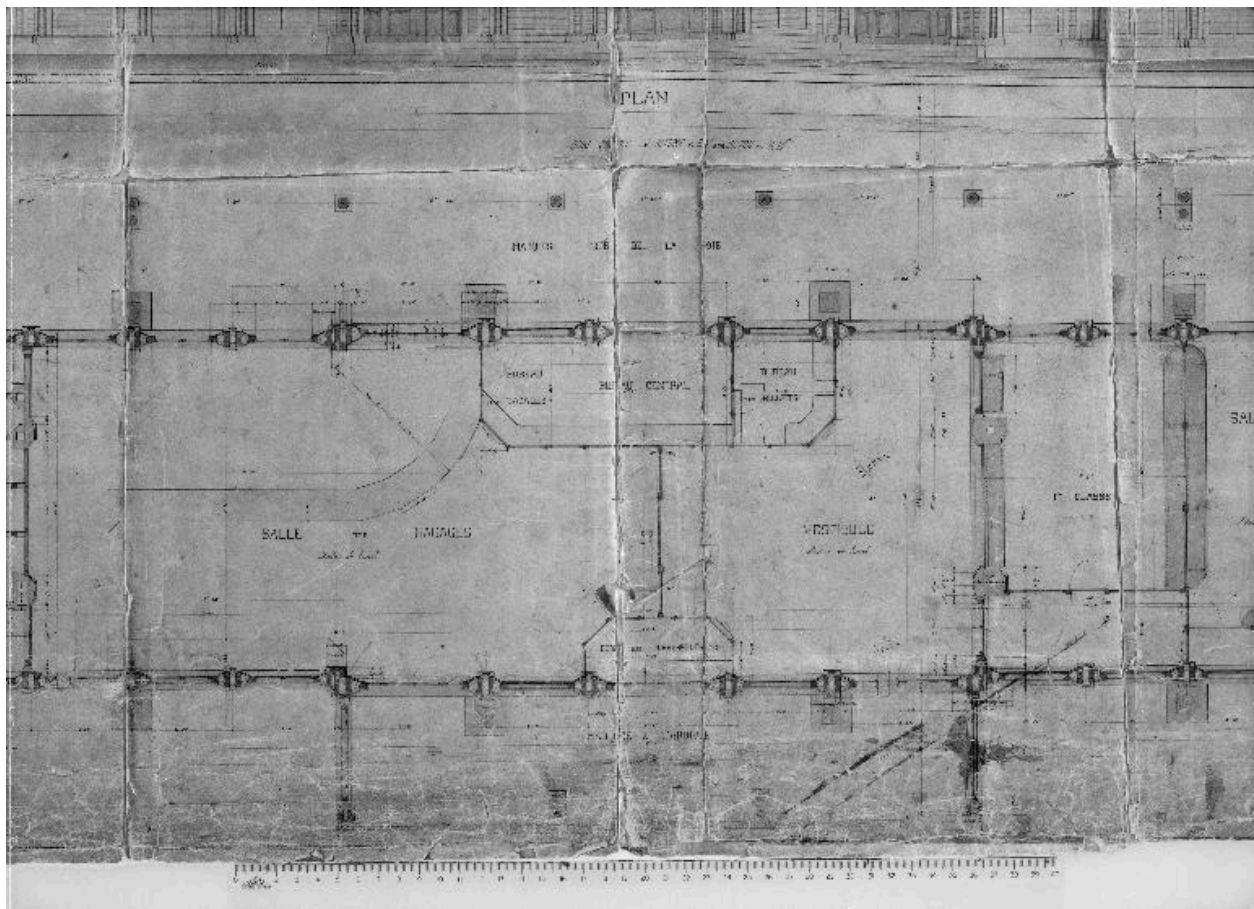
Bâtiment des voyageurs de la gare d'Abbeville, plan, détails, encre et lavis sur papier, 1857 (AC Abbeville).
