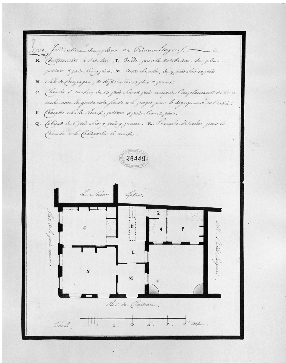
Plan du 1er étage. B.M. Boulogne-sur-Mer, 13e portefeuille, fol. 18.
