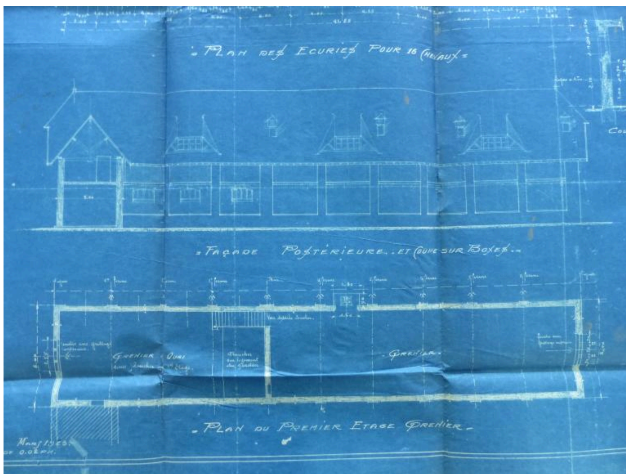
Propriété de Melle Poiret. Villers-Bretonneux. Ferme Lefèvre, route de Péronne. Construction du bâtiment des écuries. Façade postérieure et plan de l'étage, par A. Duchène, M. Dupré et M. Gauderon architectes (AD Somme ; 10R 1274).
