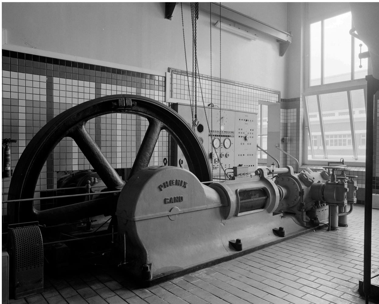
Compresseur à ammoniac Phoenix (Gand).
