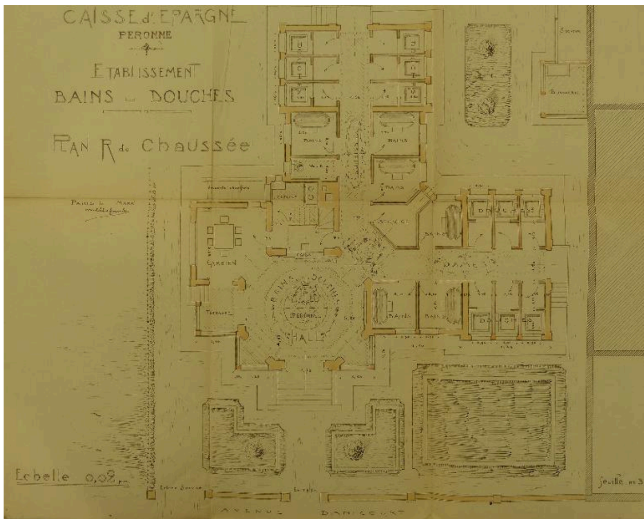
Caisse d'Epargne de Péronne. Etablissement de bains douches. Plan au sol, Marcel Debefaudé entrepreneur, 1924 (AD Somme ; 10R 1018).
