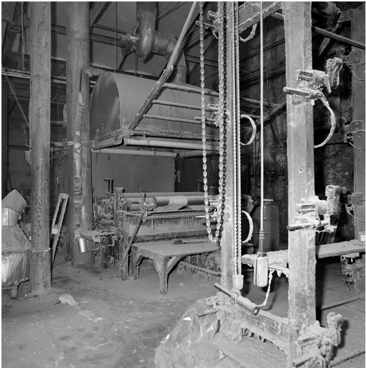
Préparation avant tissage. Encolleuse (Joseph Hibbert & Company, Darwen (GB)).
