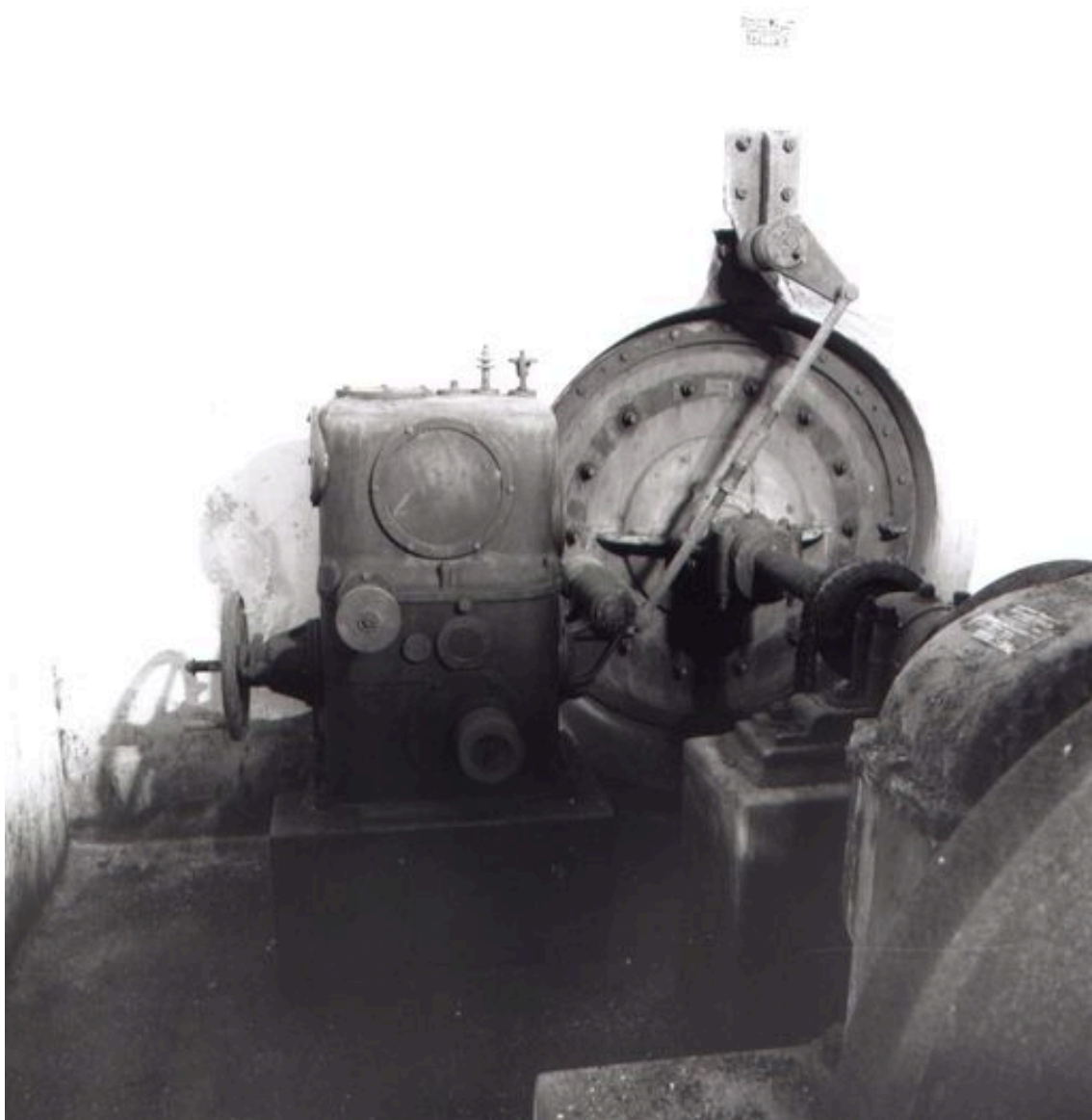
Détail de l'arbre de transmission horizontal et du régulateur.
