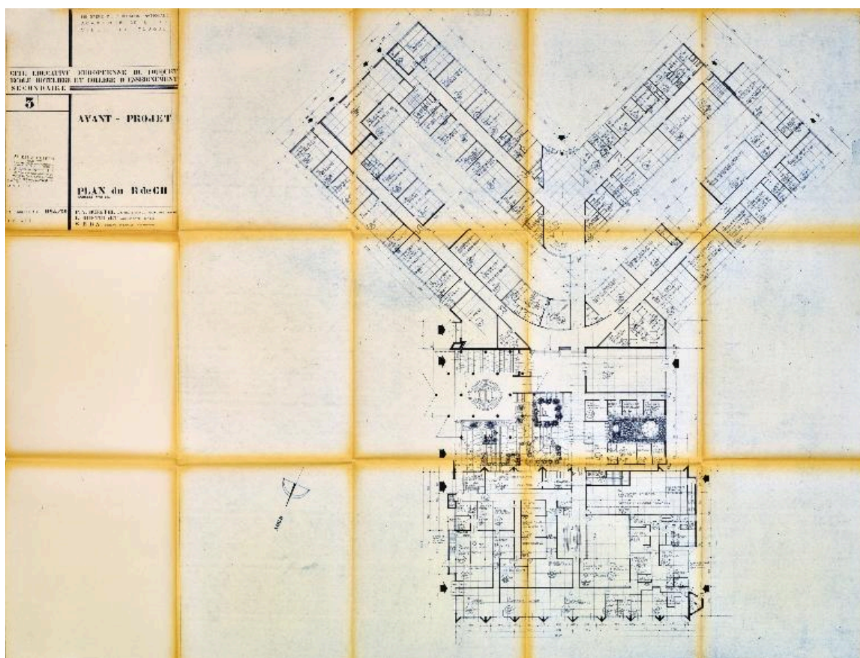
Plan de rez-de-chaussée, Avant-projet, par Pierre-André Dufétel et Louis Quételart, 1969 (AD 62 : Fonds Quételart).
