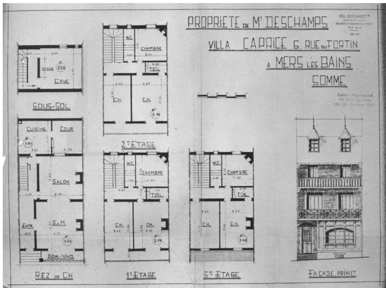
Plans de la villa Caprice (AC Mers-les-Bains).
