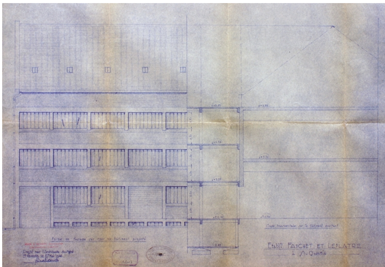
Façade sur cour du projet d'extension des ateliers de 1931, par Richard, 1946 (AC Saint-Quentin).
