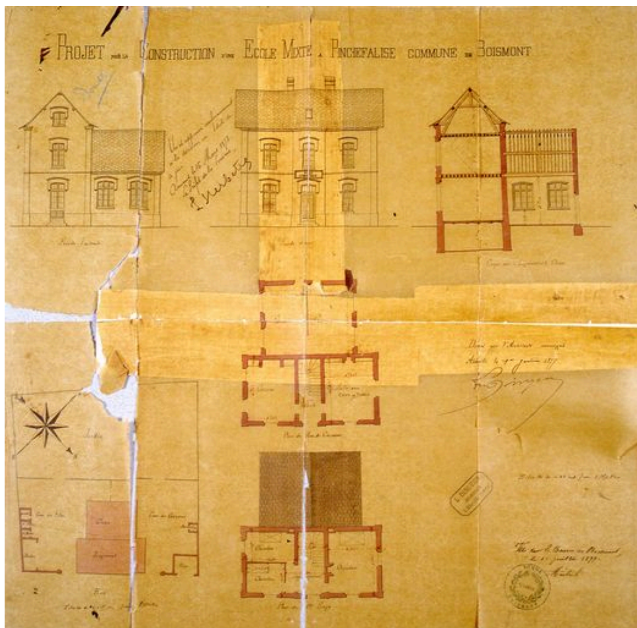
Plan, coupe et élévation du projet de l'école de Pinchefalise en 1877.
