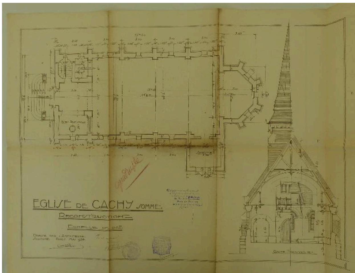
Eglise de Cachy (Somme). Reconstruction. Plan au sol et coupe latérale, Louis Duthoit, 1924 (AD Somme ; 99 O 879).
