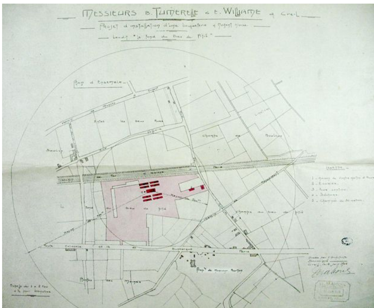
Usine III : Plan de la briqueterie Williams et Tumerelle, par Mahon, 1908 (AD Oise ; 5Mp2519).
