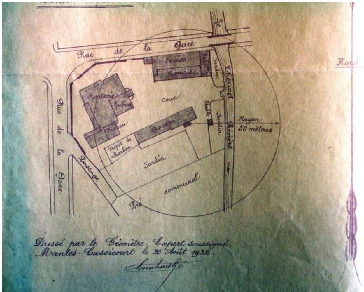
Plan masse de la laiterie, 20 août 1932.
