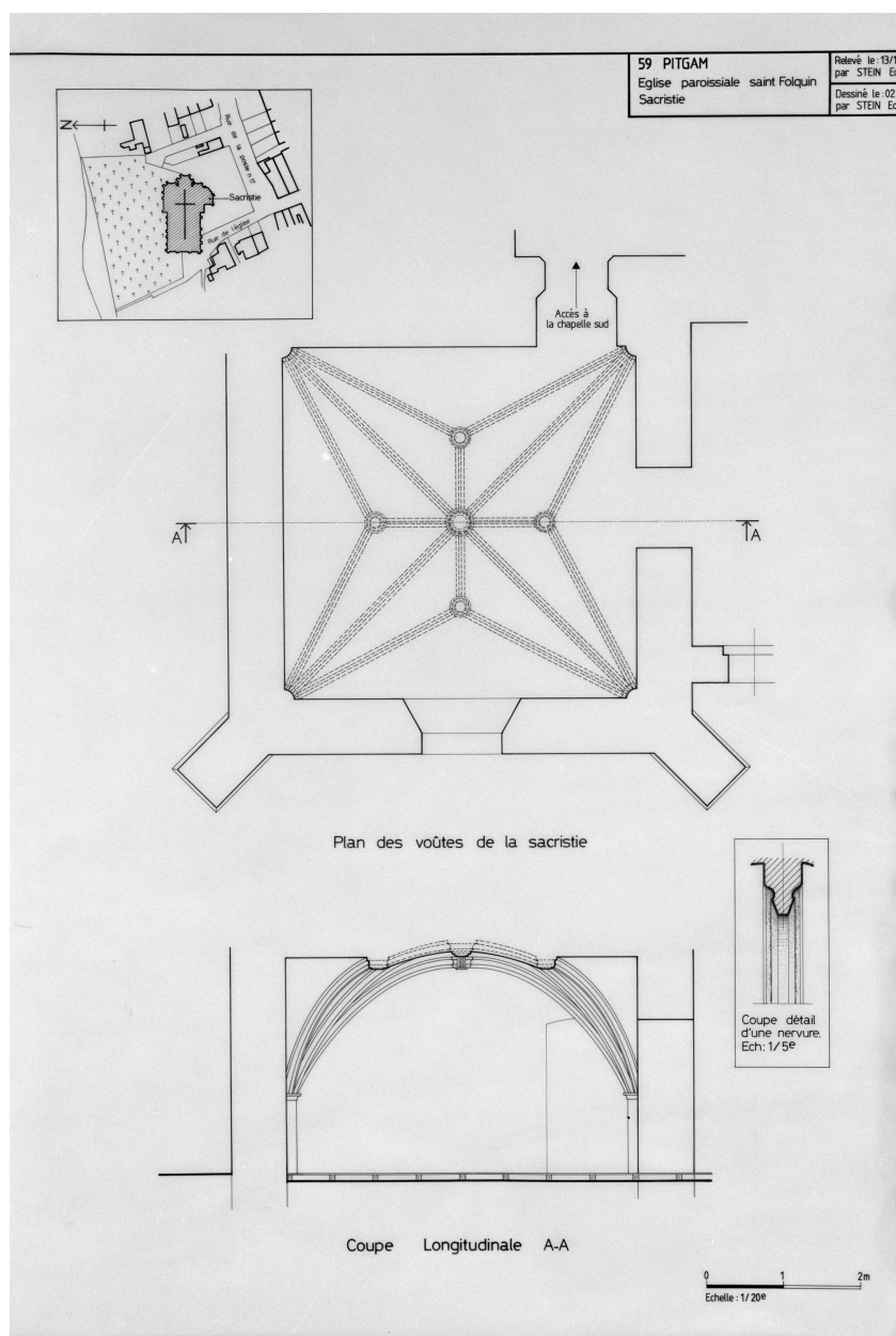
Sacristie : plan de situation, plan et coupe par Eddy Stein.
