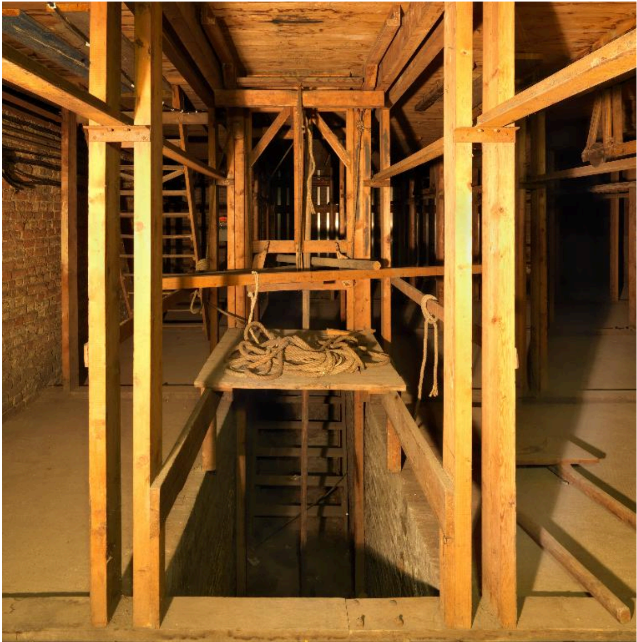
Dessous de scène, mécanisme de la trappe.
